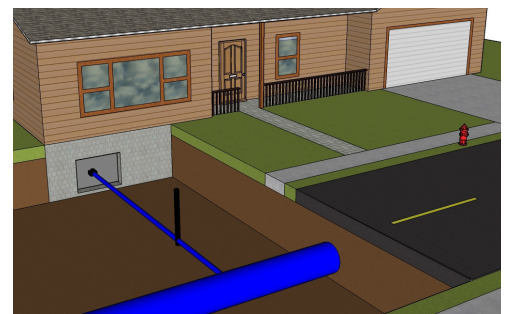
Ubicación del lateral (tubería azul pequeña) ingresando a la casa desde la tubería principal localizada a la mitad de la calle
